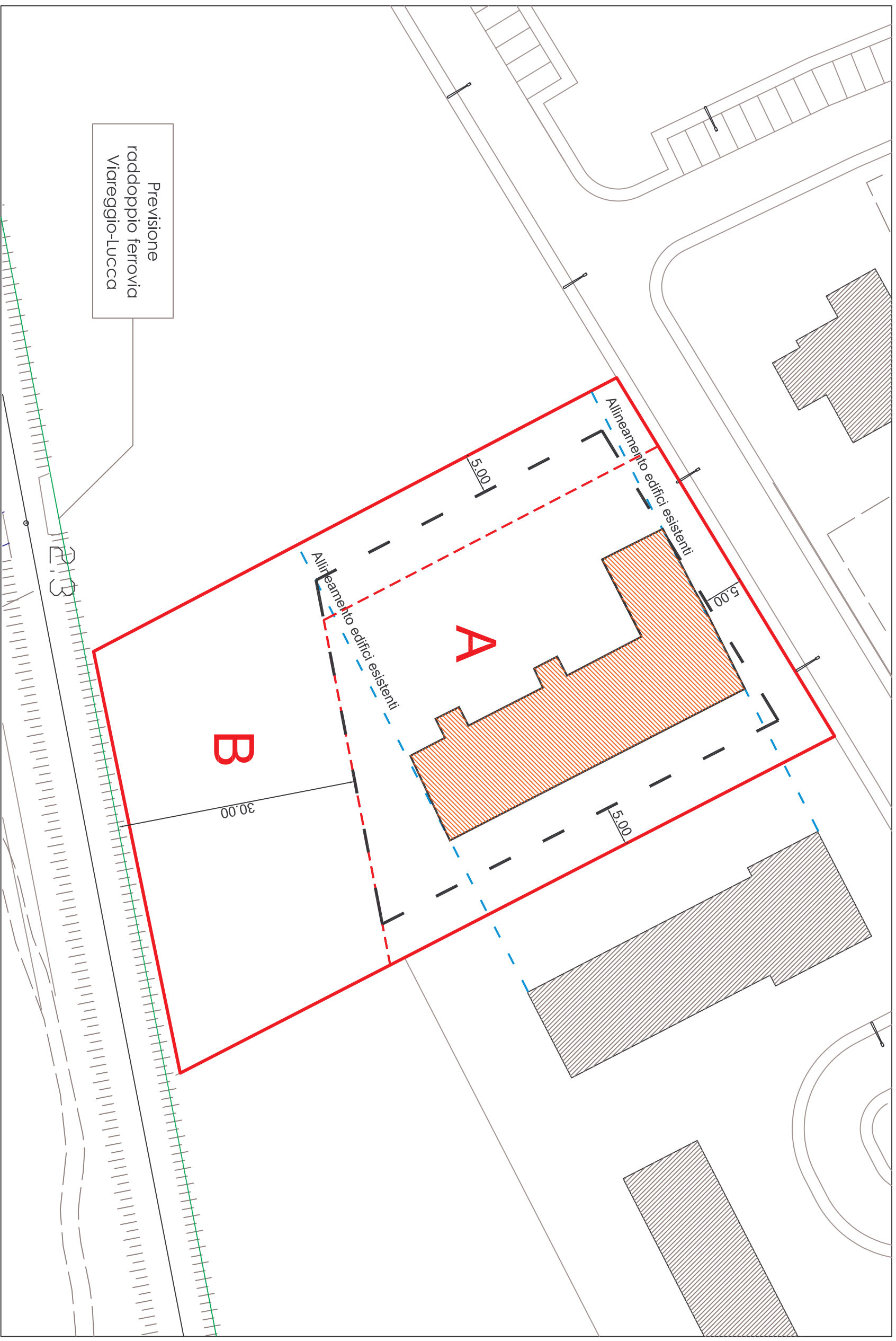
Distanze ed allineamenti 1:500
